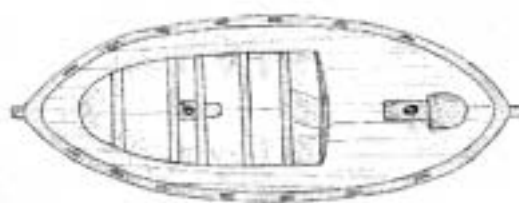
VOLANTEIRA: ESLORA, 11'55 M.; MANGA, 3'78 M. E PUNTAL, 1,80 M.
